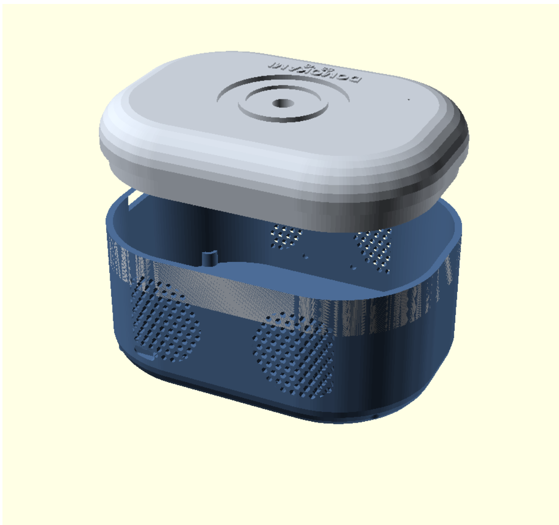
Fig. 5 - Vue éclatée du boîtier v5 : capot a molette + bac (2 HP facade, 2 radiateurs arriere).
